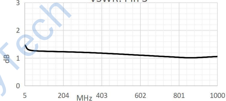
VSWR: Pin 3
