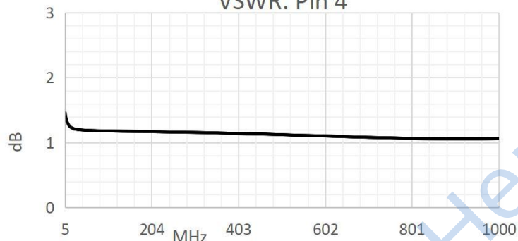
VSWR: Pin 4
