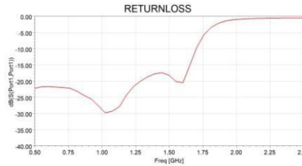
RETURNLOSS
